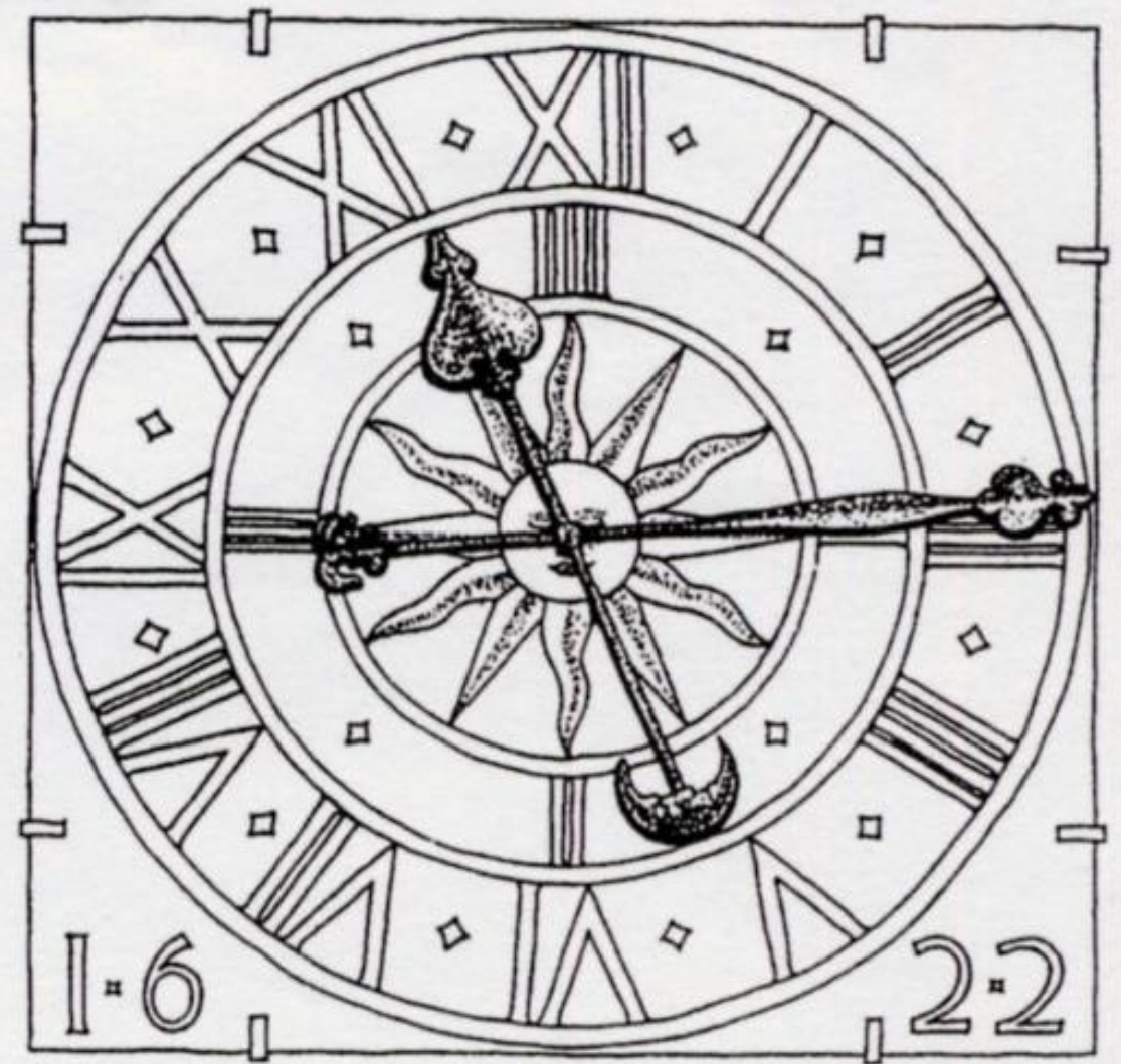
6. Szkic przedstawiający wygląd zewnętrzny tarczy zegara zamkowego. Rys. Barbara Paduch 17 / External view of the clock's face. Drawing by Barbara Paduch
